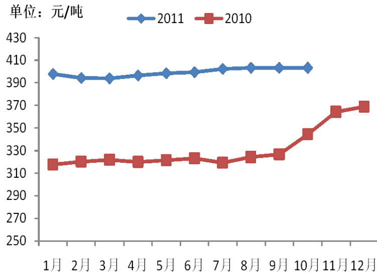
2011年全国P.0425级水泥平均价格监测
