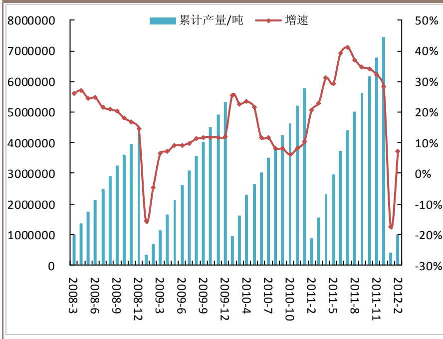
起重设备产量及同比（截止2012年02月）
