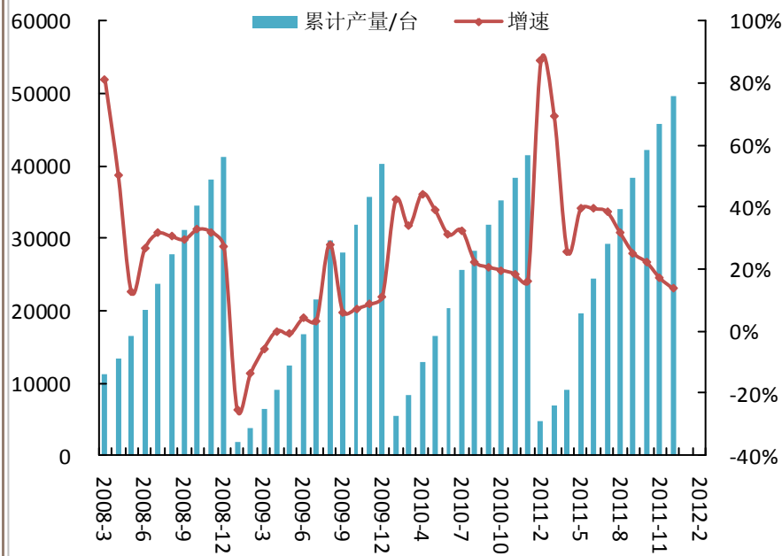
棉花加工设备产量及同比（截止2012年02月）
