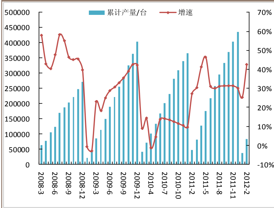
混凝土机械产量及同比（截止2012年02月）
